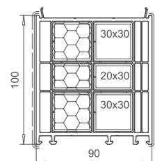
Verbreiterung 100mm 114.207 Stahl 113.025 113.019
